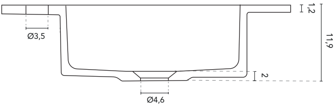
SECCIÓN
